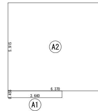
2階 床面積求積図 S:1/150
